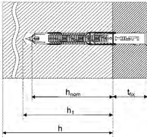
Abbildung 1: Verankerung im gerissenen und ungerissenen Beton
