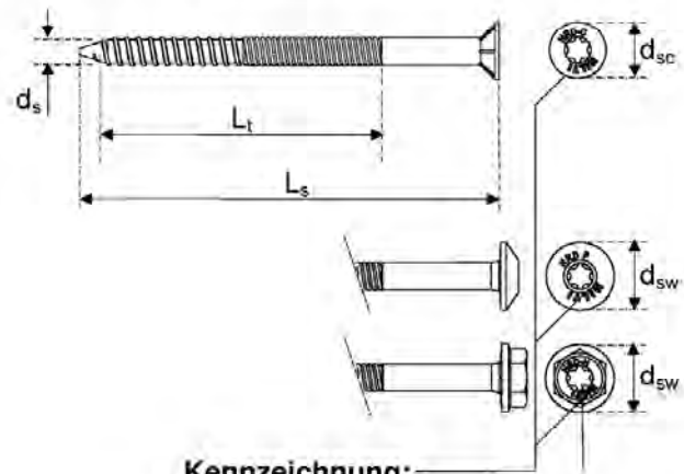
Abbildung 3: Spezialschraube
