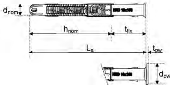
Abbildung 2: Kunststoffhülse
